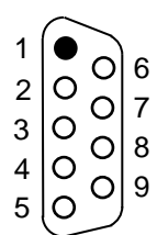
Вилка DB-9M («Папа») Вид со стороны монтажа
