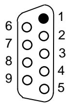
Розетка DB-9F («Мама») Вид со стороны монтажа
