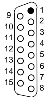
Розетка DB-15F («Мама») Вид со стороны монтажа
