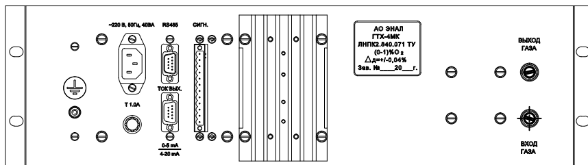
Общий вид газоанализатора ГТХ-4М
