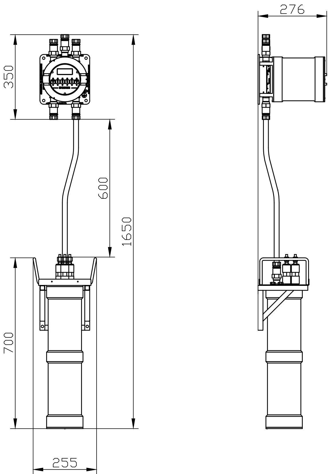
Общий вид газоанализатора EN2000B
