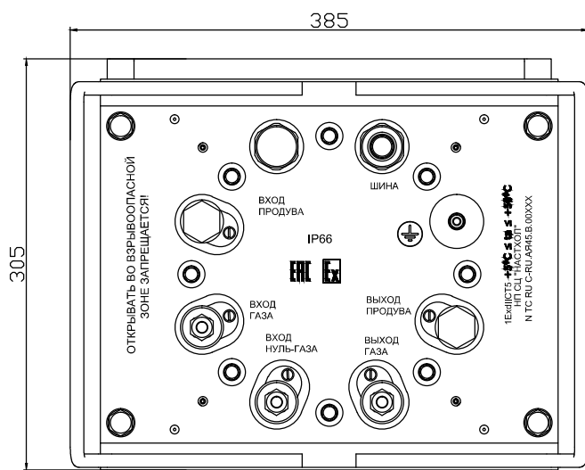
Общий вид преобразователя EN700B
