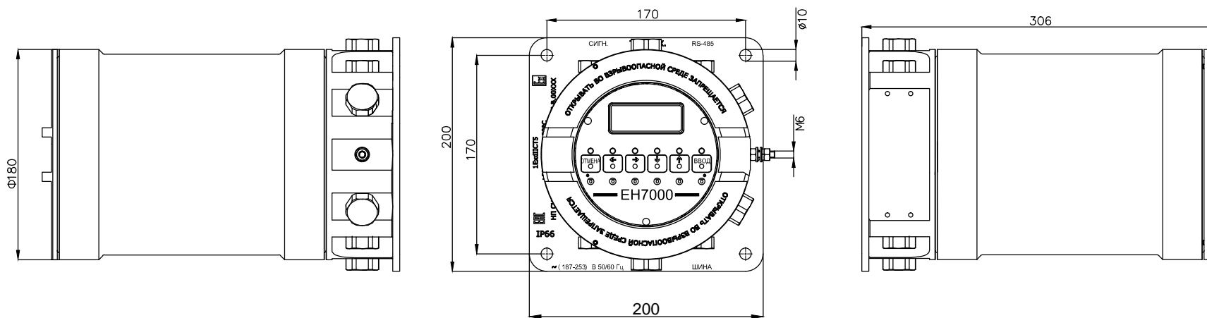
Общий вид блока вторичного преобразователя БВП-3В
